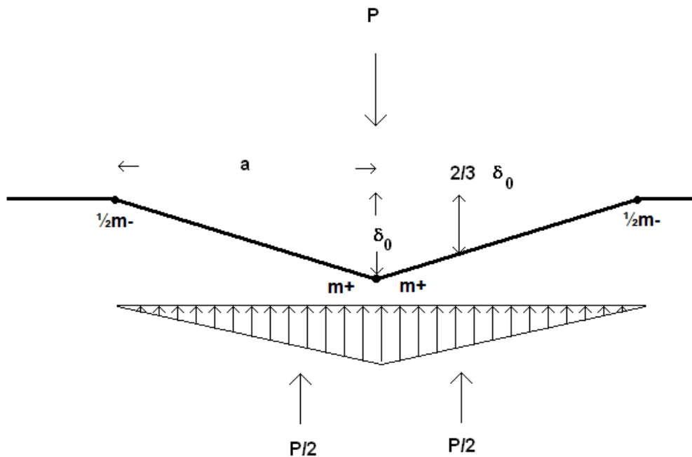
Figur 4. Ligevægt
