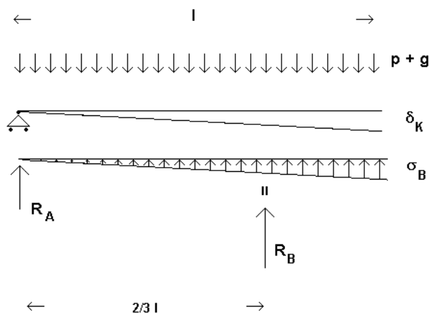
Figur 6. Spændingsfordeling
